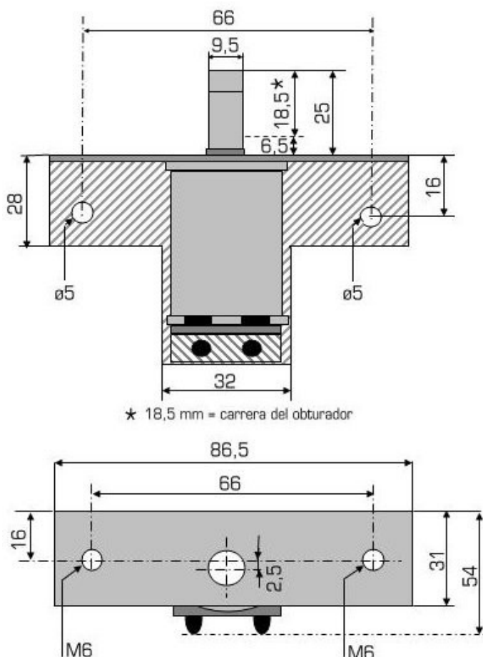
CÓDIGO EI-05-110 Mecanismo obturador universal completo 110 VAC
